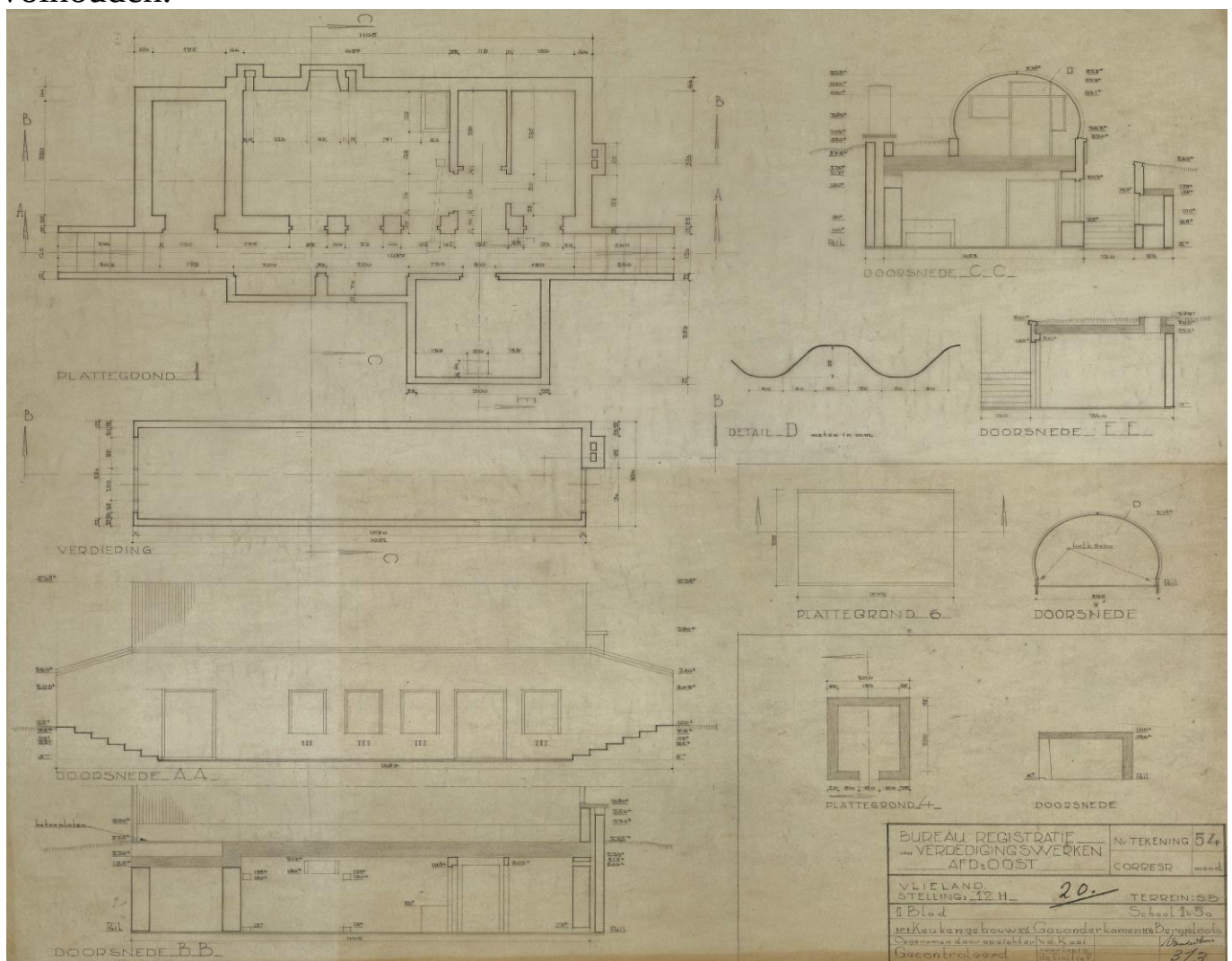
Tekening keukenbunker Stelling 12H
