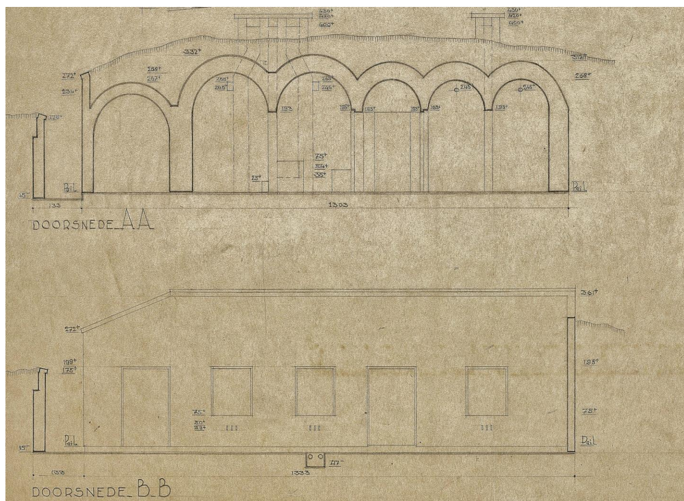
Tekening keukenbunker Stelling 13H
